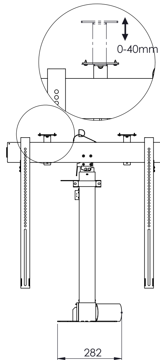
SZCZEGÓŁ D SKALA 1 : 5
